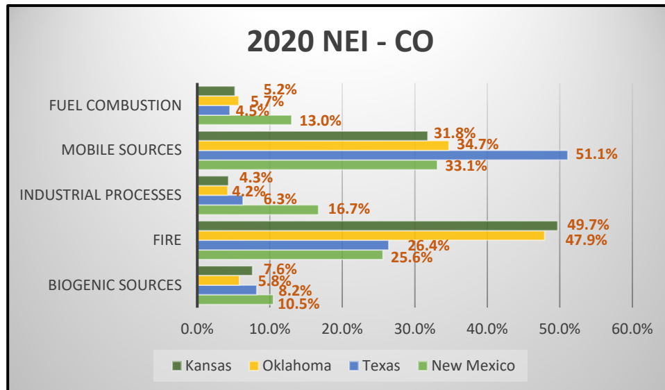
Figure 5. 2020 NEI – CO.
